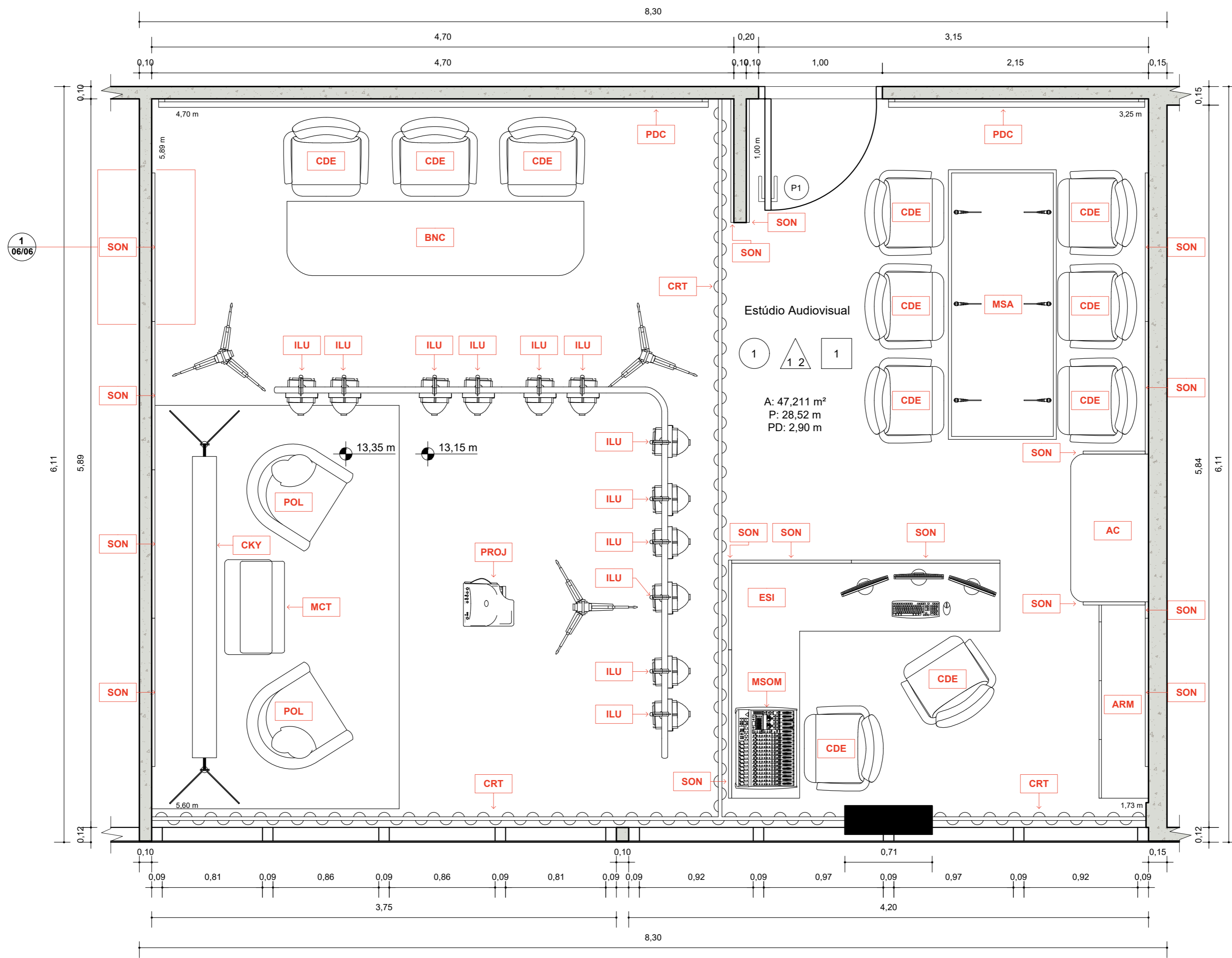
3 PLANTA BAIXA - LAYOUT ESCALA 1:25
